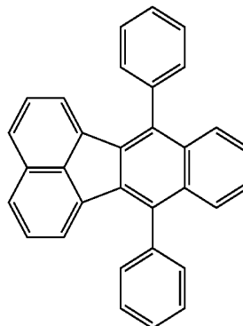
7,12-Diphenylbenzo[k]fluoranthene
